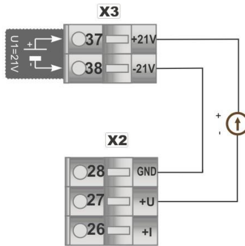
Рисунок Б.2 - Подключение к индикатору ИТМ-111 аналоговых датчиков с пассивными выходами
